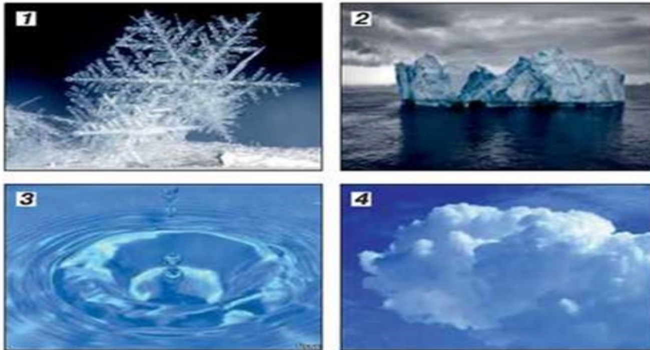
Мал. 31. Агрегатні перетворення води
